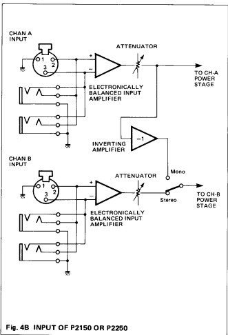
Fig. 4B INPUT OF P2150 OR P2250
